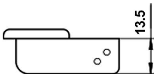
глубина чашки 13.5
